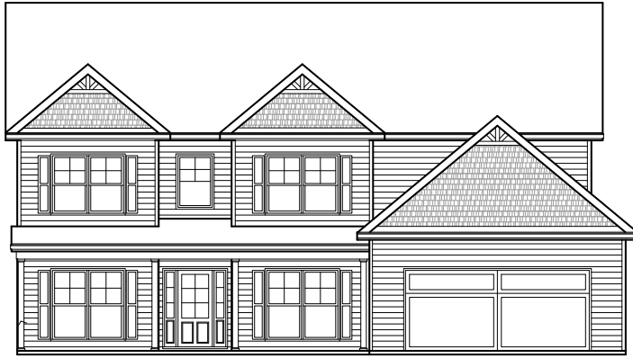
ELEVATION A
